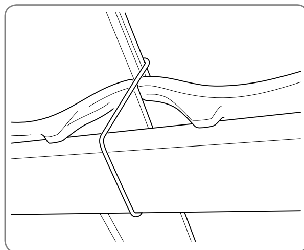
Fastgørelse med en sidefalsbinder, som fastgøres til tagstenens sidefals.
