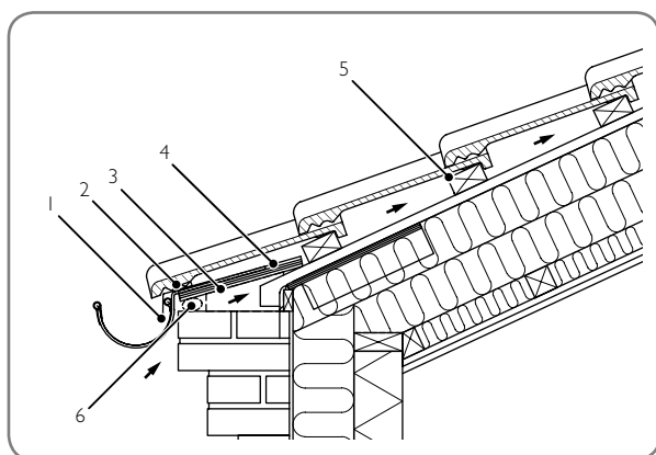
Montering af tagfod med B&C Danflock ved gesims: 1. Fodblik, 2. Fugleklo, 3. Underlag for fodplade, 4. Fodplade, 5. Lægte, 6. Snefangsrør.
