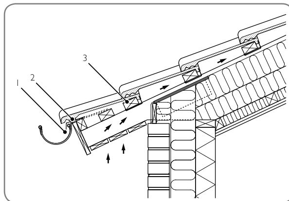
Montering af tagfod med B&C Danflock ved udhæng: 1. Fodblik, 2. Fugleklo, 3. Lægte.
