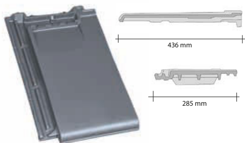
Udluftningssten, Vægt: ca. 4,1 kg
