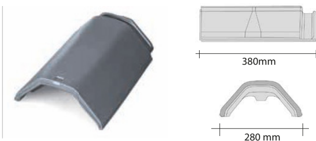
Rygning Vægt: ca. 4,4 kg
