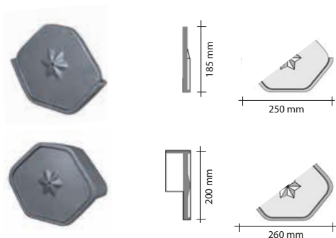
Rygning, start/slut Vægt: ca. 0,95 / 1,64 kg
