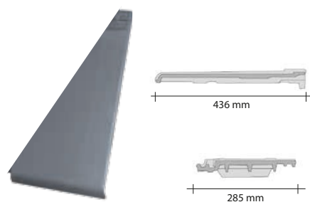
Standardsten: Vægt: ca. 3,95 kg Forbrug/m 2 : ca. 11,8 - 12,8 stk.
